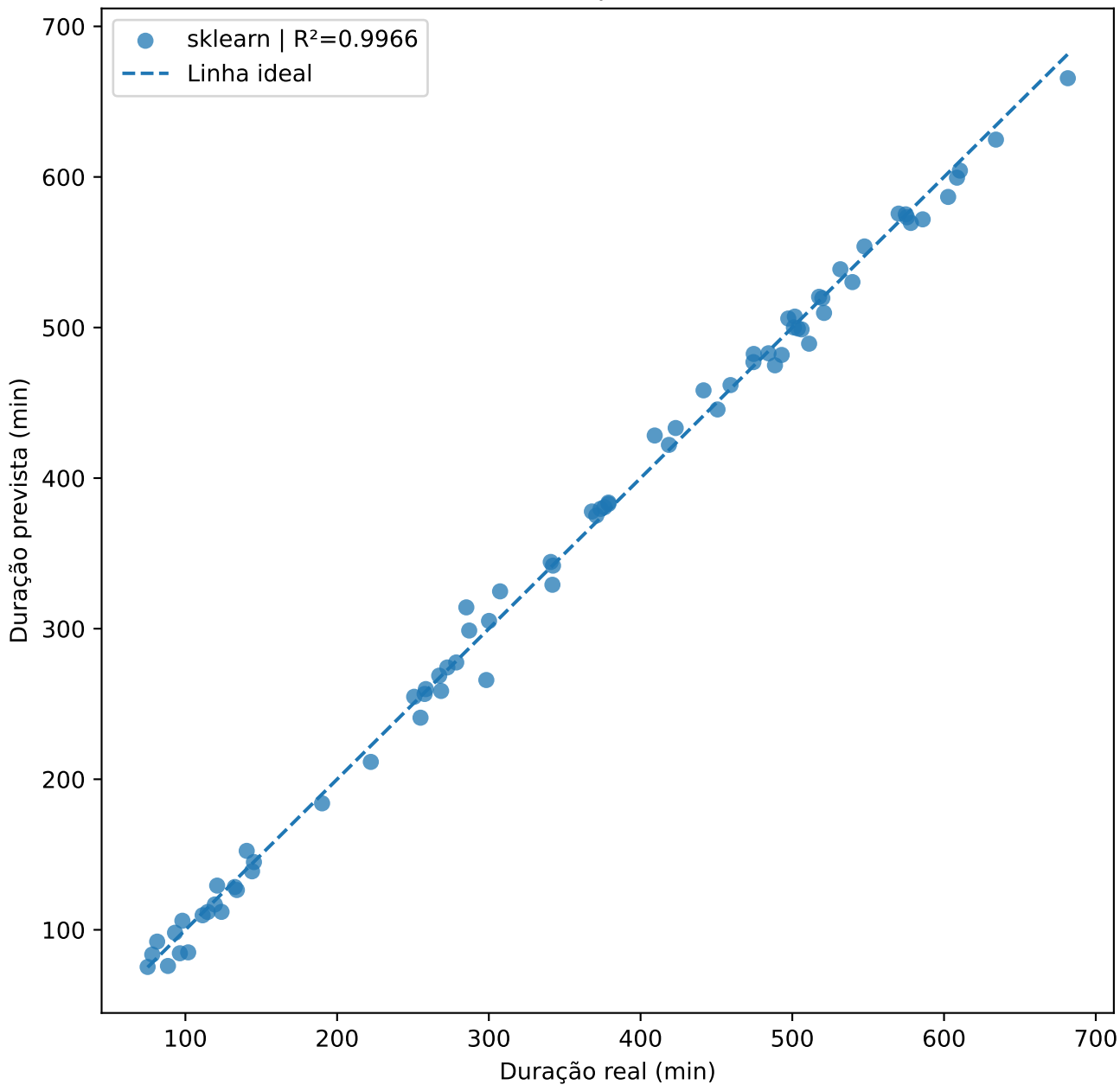
Valores reais vs. previstos - sklearn
